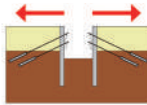
壁が倒れないようケーブルを引っ張る
